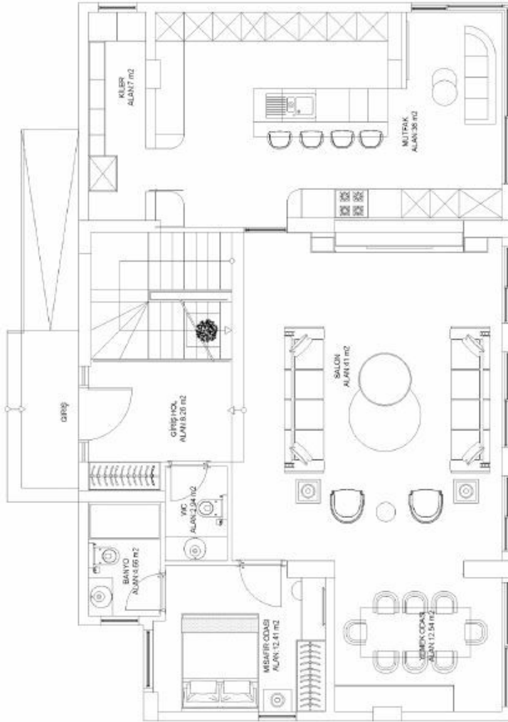
ZEMİN KAT PLANI
